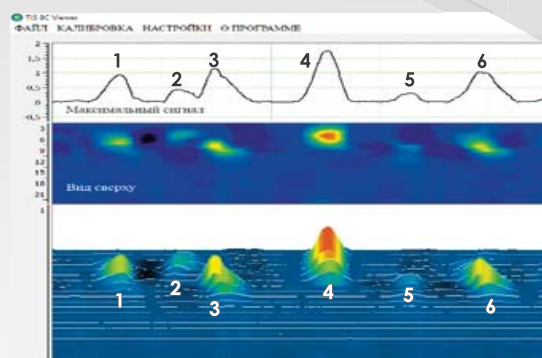
Пример обнаружения коррозионного повреждения на внутренней поверхности стенки трубопровода
