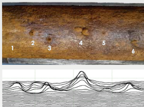
Пример обнаружения коррозионного повреждения на внутренней поверхности стенки трубопровода
