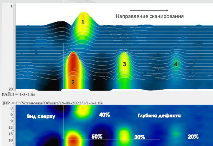
Пример обнаружения коррозионного повреждения на внутренней поверхности стенки трубопровода
